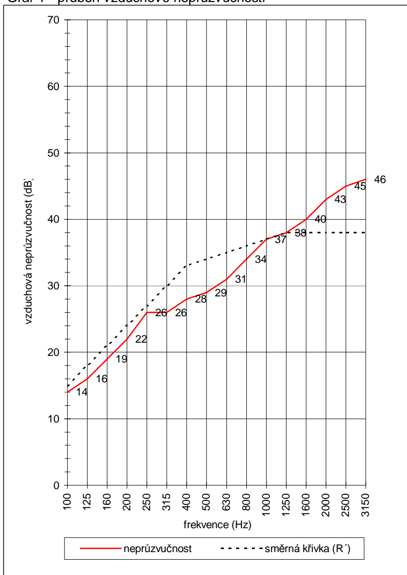
Graf 1 - průběh vzduchové neprůzvučnosti
